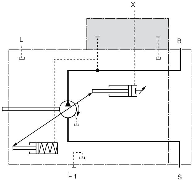
油路图
