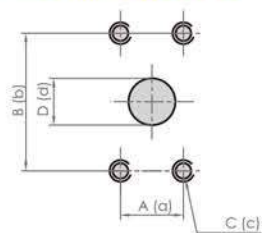
PF (G, BSPP)
