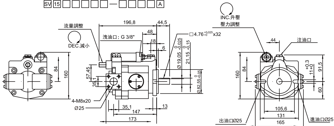
SV15A, SV18A 標準型壓力控制 (SAE A 兩孔型, 需特別註明訂購碼加A)
