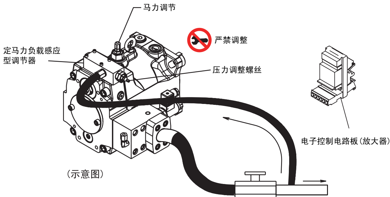
定马力负载感应型调节器+比例流量+溢流阀 PQ
