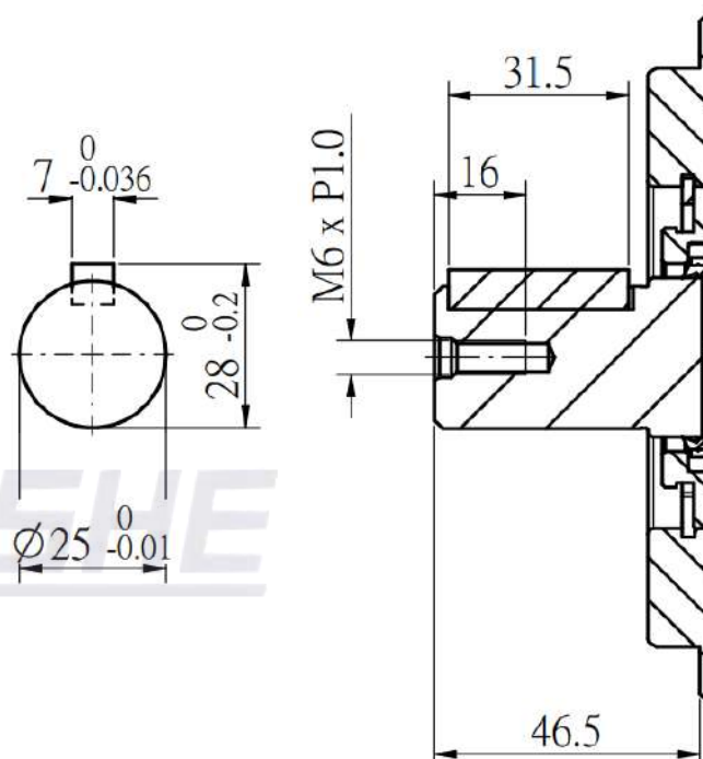
K3 : 直鍵軸 25*7*7
