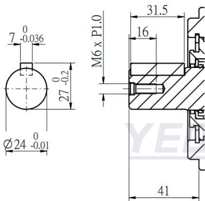
K1 : 直鍵軸 24*7*7
