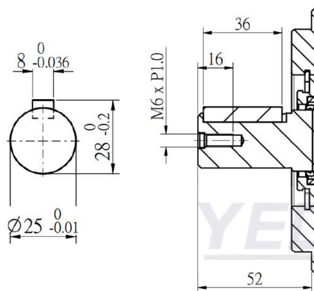
K4 : 直鍵軸 25*8*7
