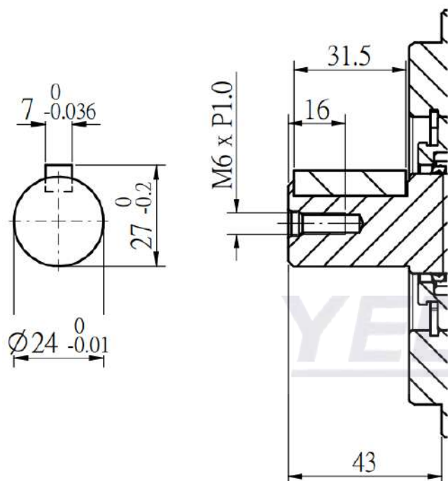
K1 : 直鍵軸 24*7*7
