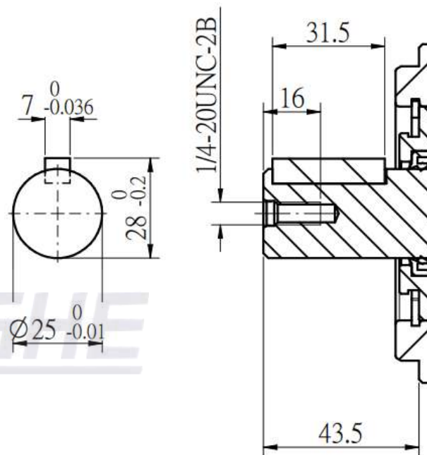
K3 : 直鍵軸 25*7*7
