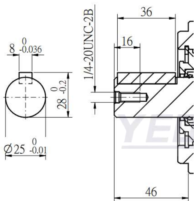
K4 : 直鍵軸 25*8*7
